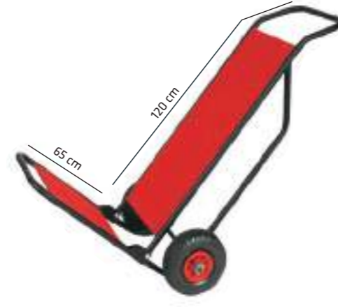
Boyalı Valiz Taşıma Arabası Luggage Carry Cart With Painted Hanger 7455
